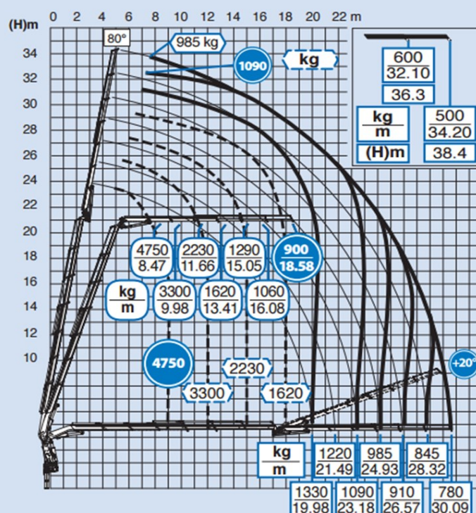
Diagramme de levage avec treuil et Jib
