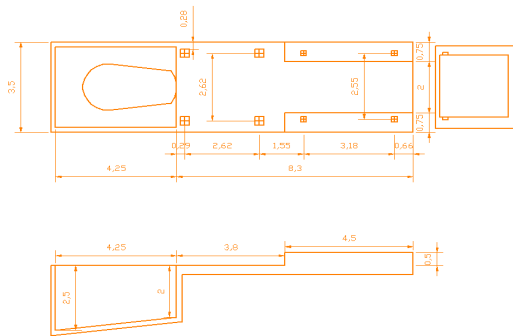
Centrale à béton GH 1000 N+S
